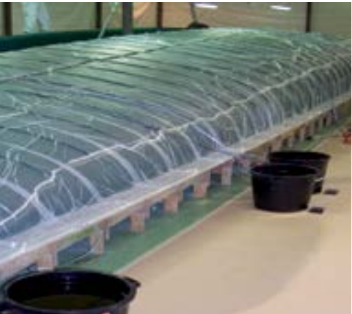
Vacuuminfusion avec Biresin® CR131.
